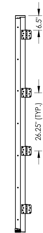
HINGE JAMB
