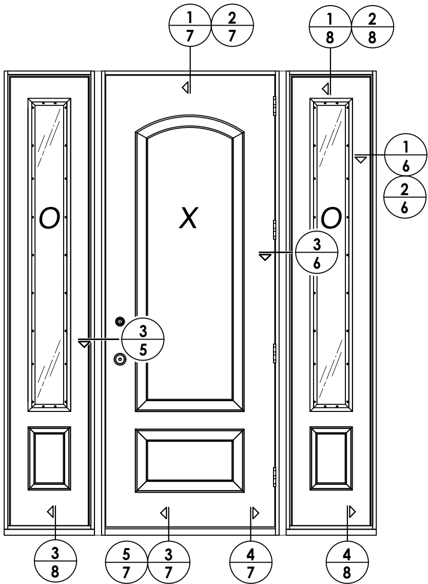
ELEVATION (OXO)
