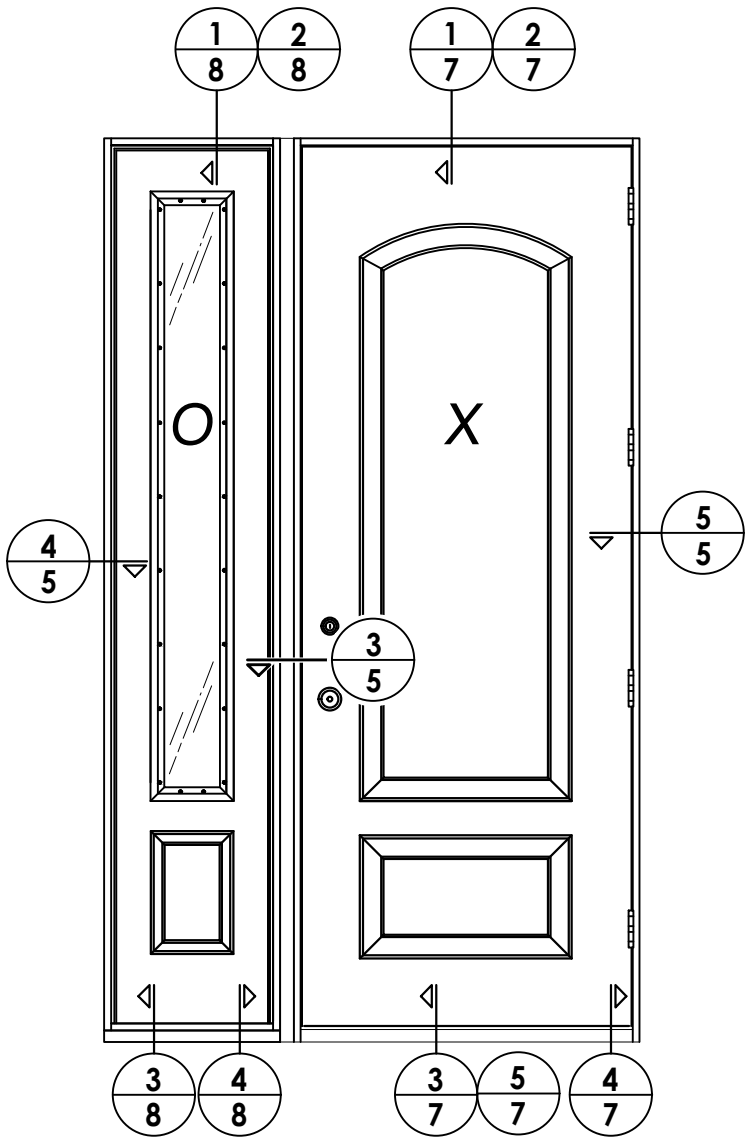
ELEVATION (OX / XO)
